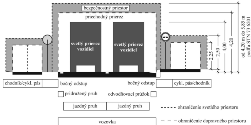
Obrázok 1 a) – Priechodný prierez MK
